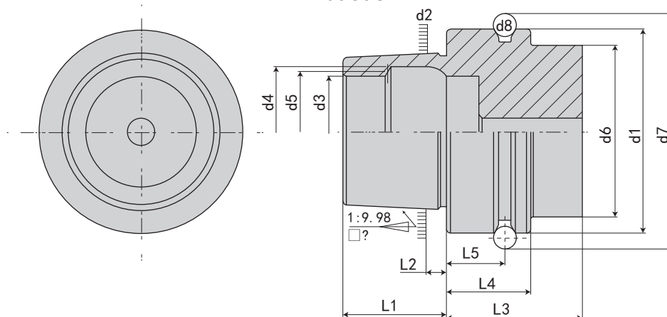
DIN 69893E
